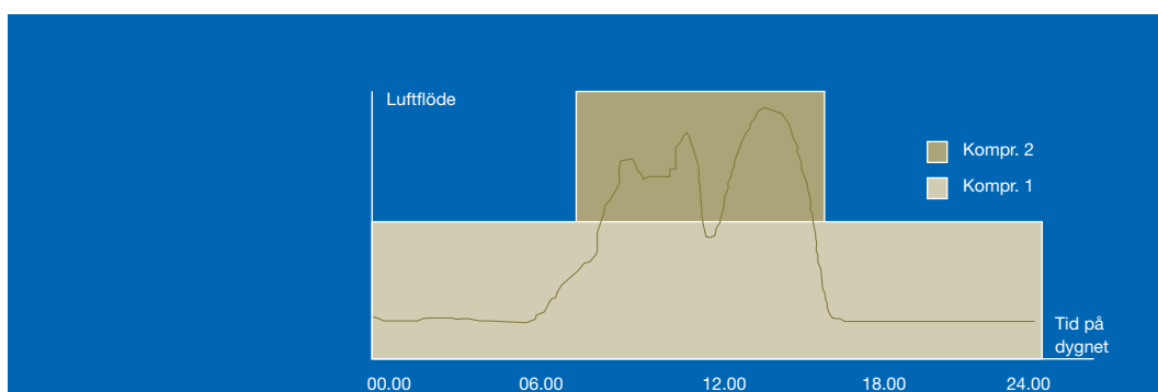
Figur 3. Två kompressorers gångtid och luftflöde under ett dygn.
